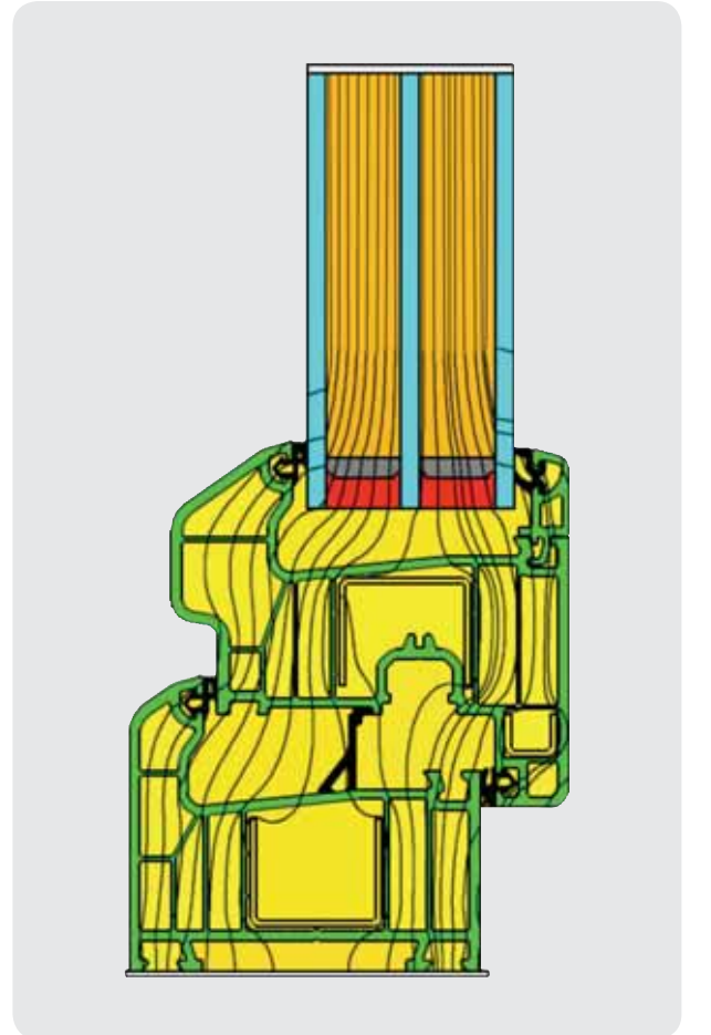
PENCERE ISI AKIŞI DİYAGRAMI UF:1,02 W/M 2 *K UW: 0,94 W/M 2 *K
