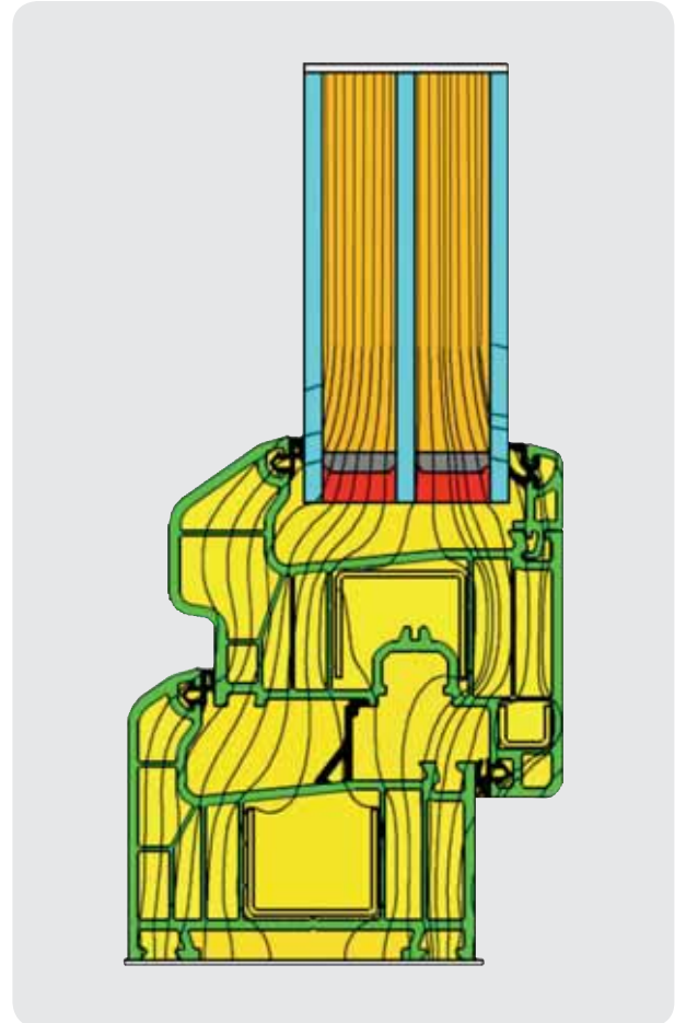
PENCERE ISI AKIŞ DİYAGRAMI UF:1,02 W/M 2 *K UW: 0,94 W/M 2 *K
